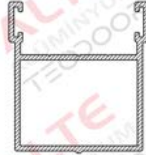
Bitiş U Profili KS - 012 440 gr/m
