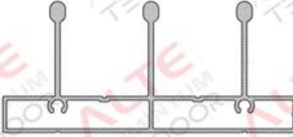
Eşki Sürme Alt Kasa KS - 009 1287 gr/m
